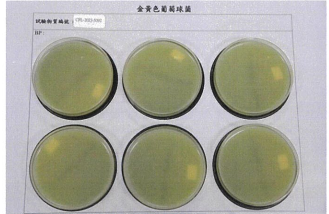
圖 1、沙門氏桿菌 XLD agar、BS agar 及 HE agar 試驗結果圖 圖 2、金黃色葡萄球菌 BP agar 試驗結果圖
